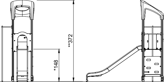
KPL101622 1:100
