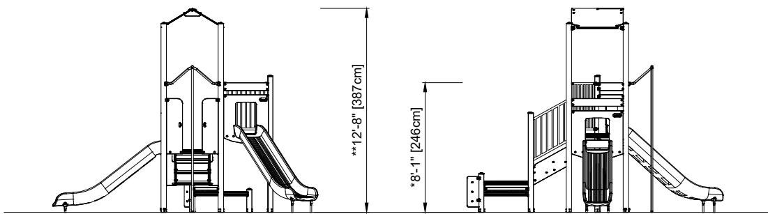
PCE 111434 1:100
