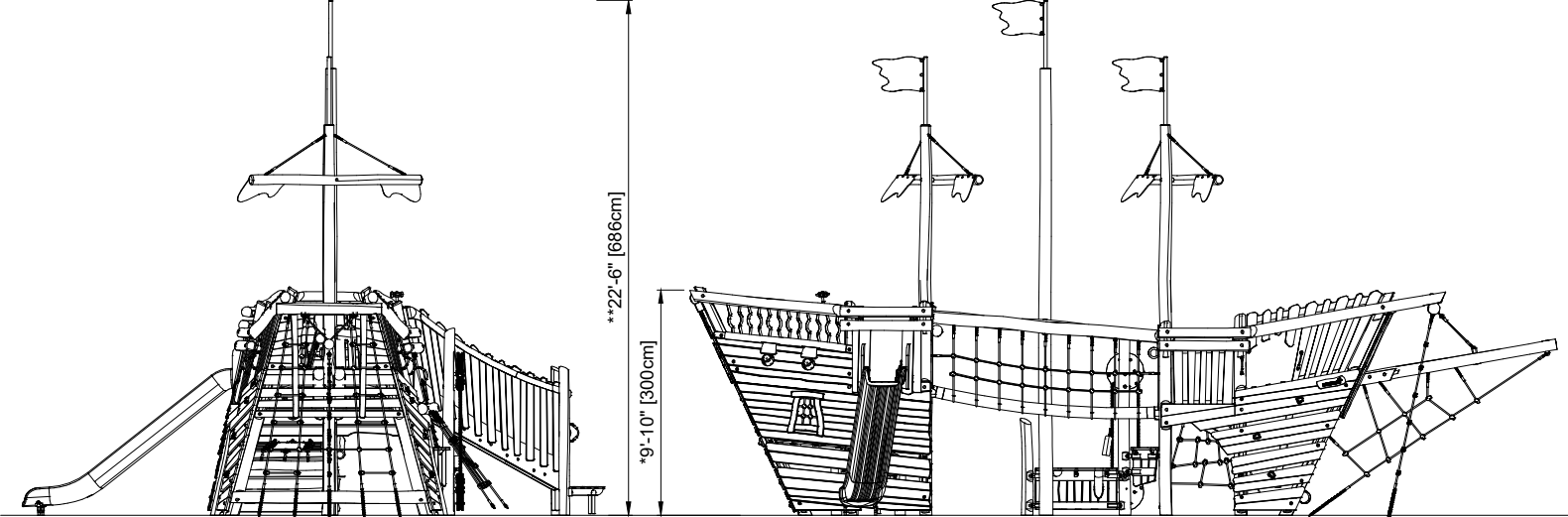
NRO545 1:100
