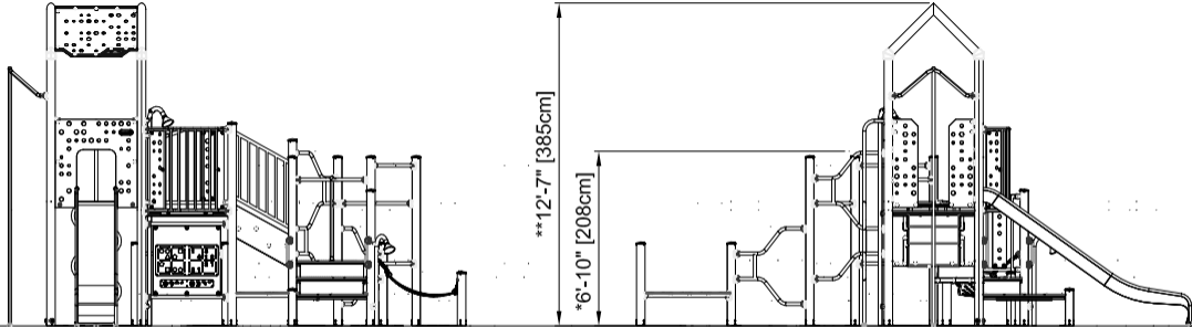
PCX210100 1:100
