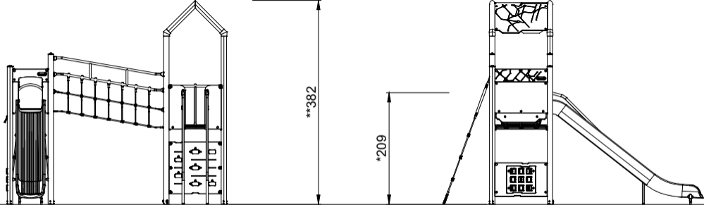
PCM212821 1:100
