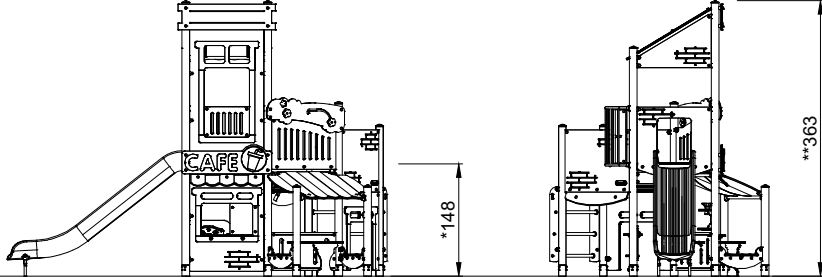
PCM52321 1:100
