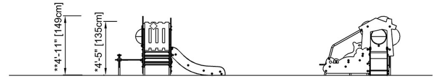
MSC541701P 1:100
