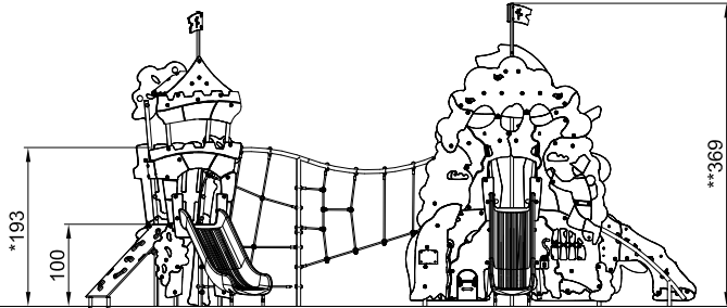
MSC643200 1:100
