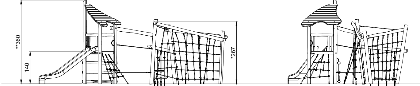
NRO1001 1:100
