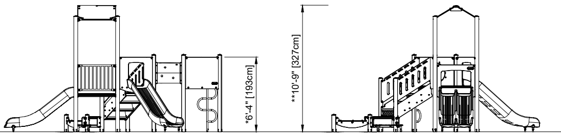
PCE205734 1:100
