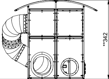
PBO100101 1:100
