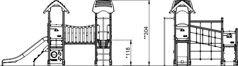
KPL400612 1:100
